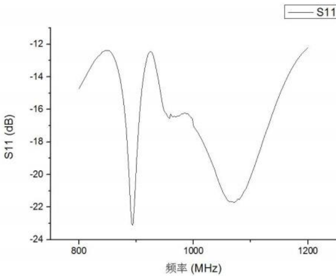
驻波测试图
