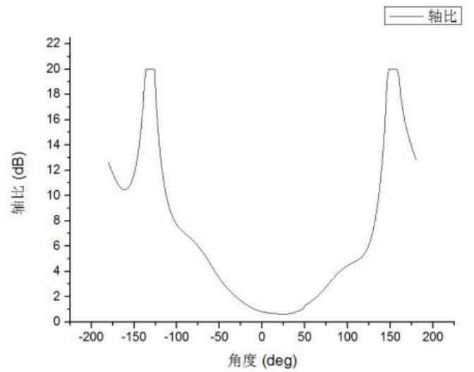
轴比测试图
